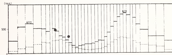
Fig-5 Maximum axial force (KUWT-3 P-2) h=0.1
